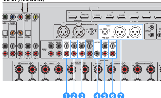
Gerät (Rückseite)
