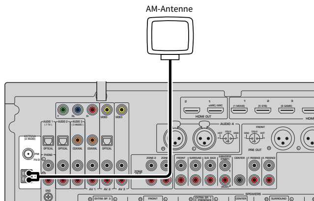
Gerät (Rückseite)
