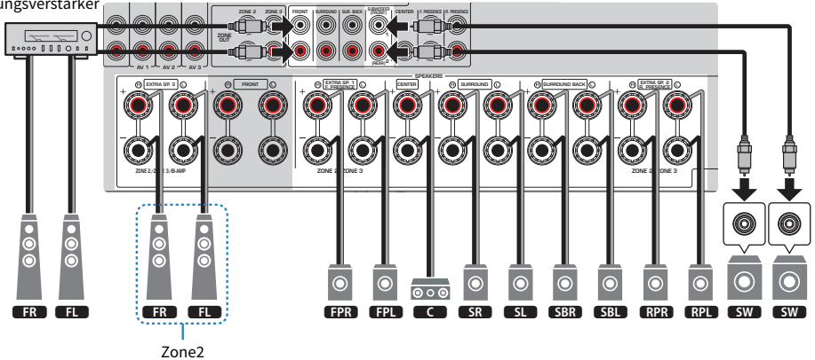
Externer Leistungsverstärker
